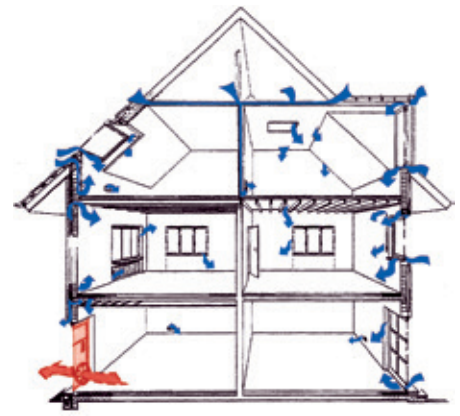
Das Messprinzip: Ein Ventilator saugt Luft aus dem Gebäude, Außenluft strömt durch Leckagen ins Innere
