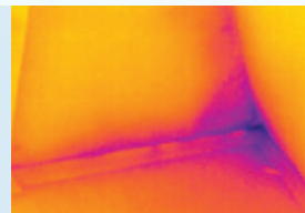
Thermogramm einer Luftleckage
