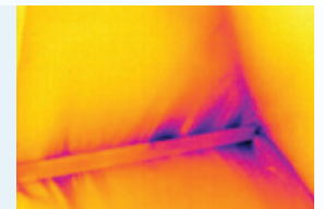
Eindeutigeres Thermogramm während des BlowerDoor Tests
